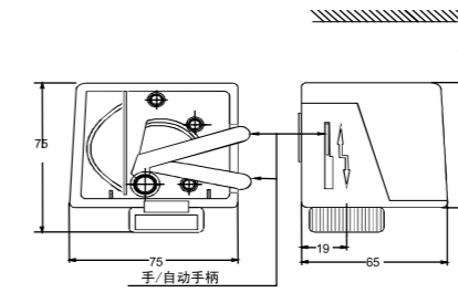
尺寸(mm)
